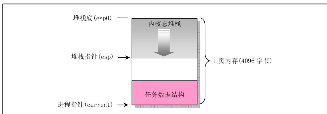
图 5-25 进程的内核态堆栈示意图
