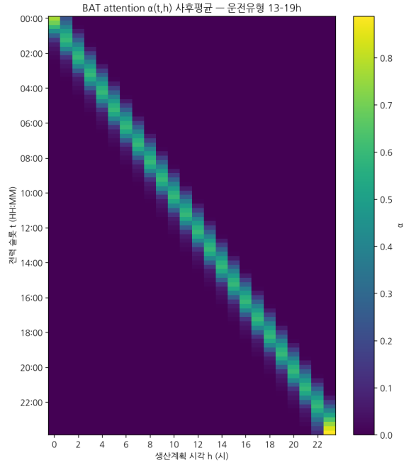
그림 1: 13-19시간 가동유형의 어텐션 가중치 \alpha_{t,h} 사후평균. 세로축은 전력 슬롯, 가로축은 생산계획 시각이다.
