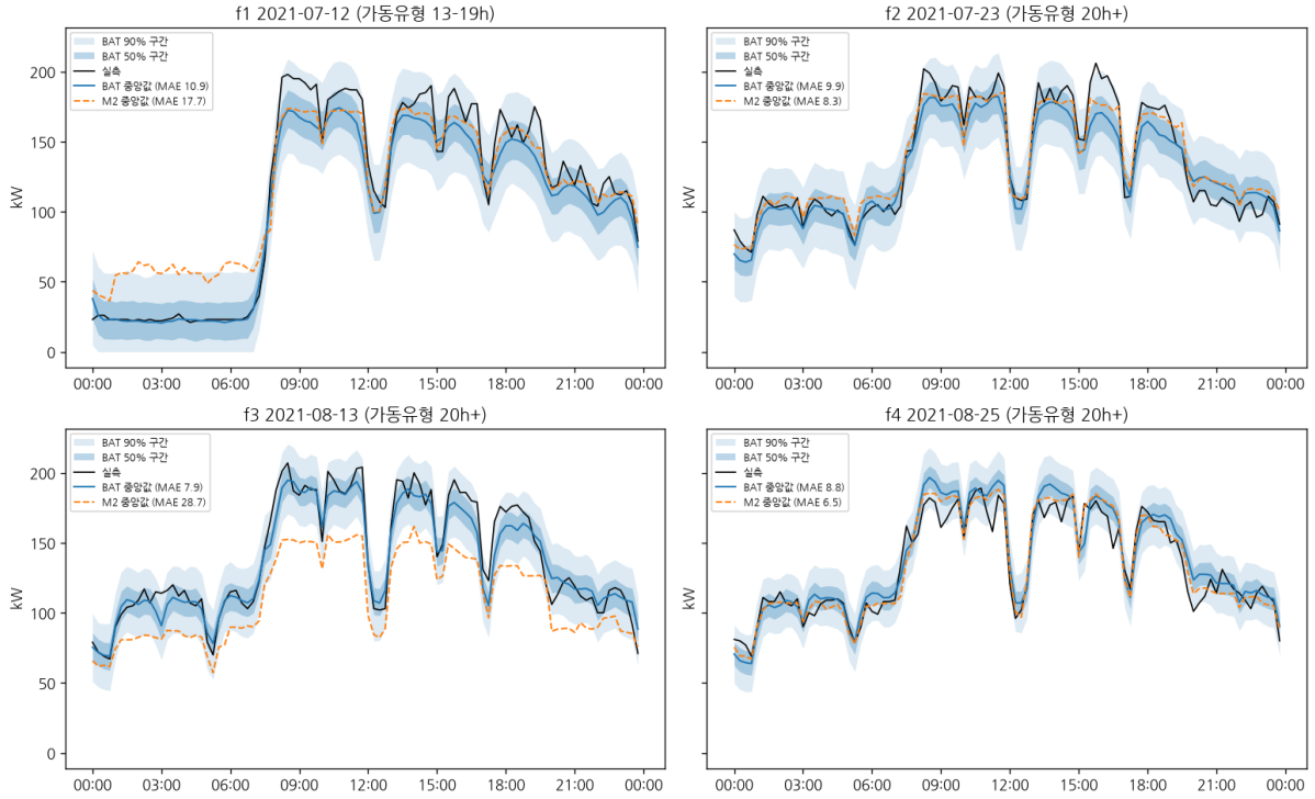
그림 1: 검증 fold별 대표일(일 MAE가 fold 중앙값에 가장 가까운 가동일)의 실측, BAT 중앙값과 50·90% 예측구간, M2 중앙값.
