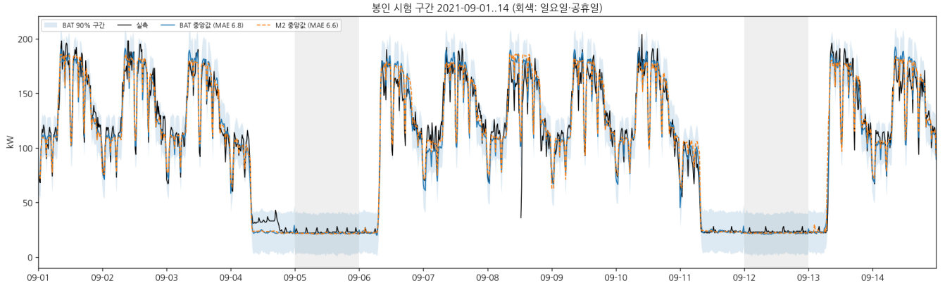
그림 2: 봉인 시험 구간(2021년 9월 1–14일)의 실측, BAT 중앙값과 90% 예측구간, M2 중앙값. 회색은 일요일이다.
