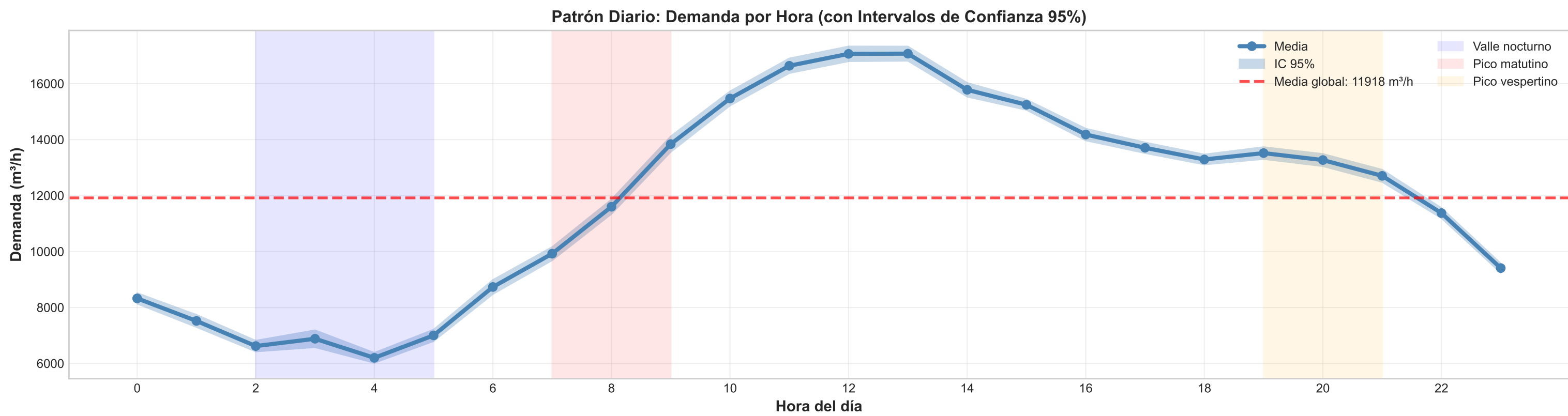
Figura 4.4: Análisis de Patrones Temporales en la Demanda de Agua
