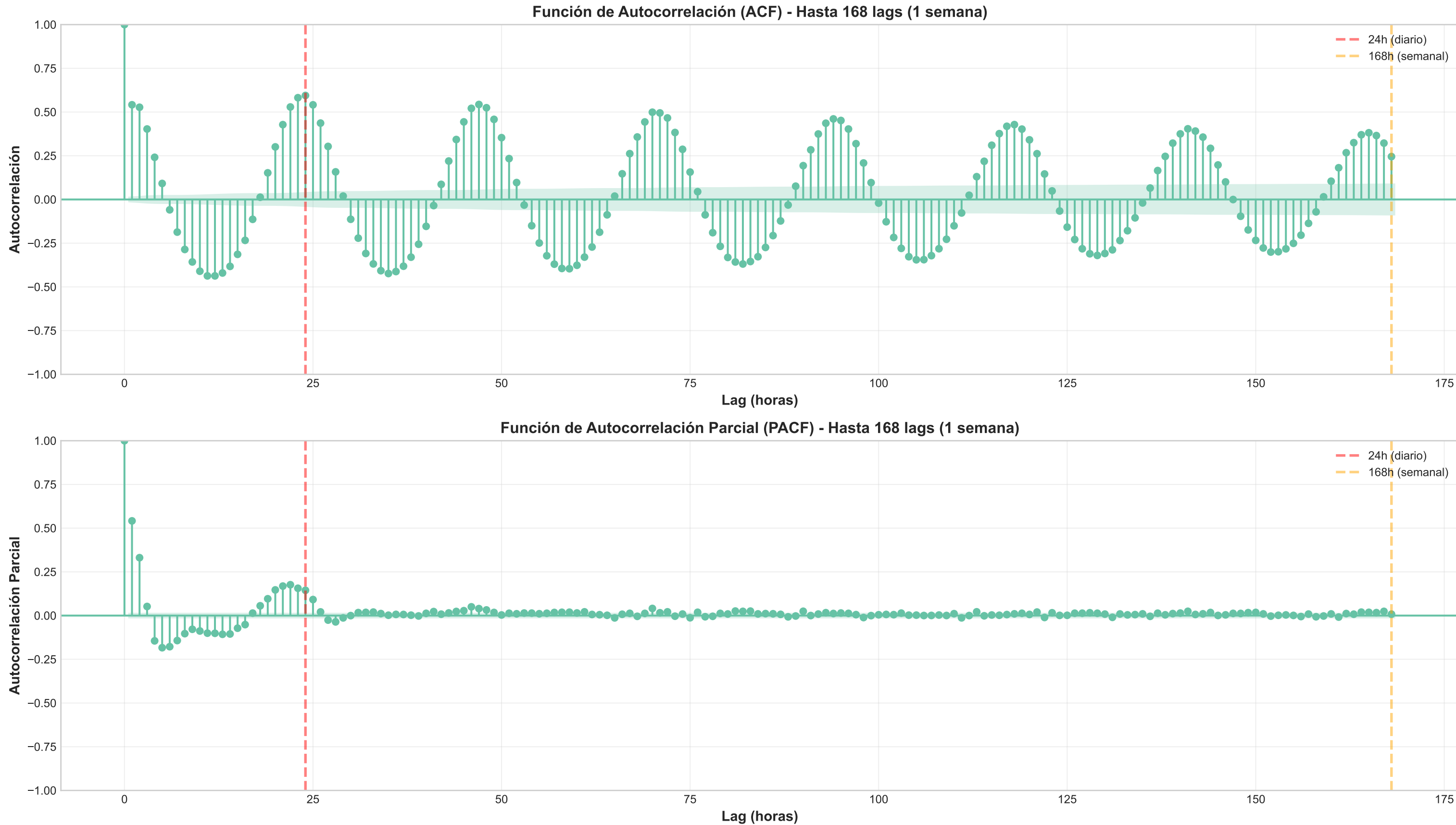
Figura 4.5: Análisis de Autocorrelación - Justificación de Modelos de Series Temporales
