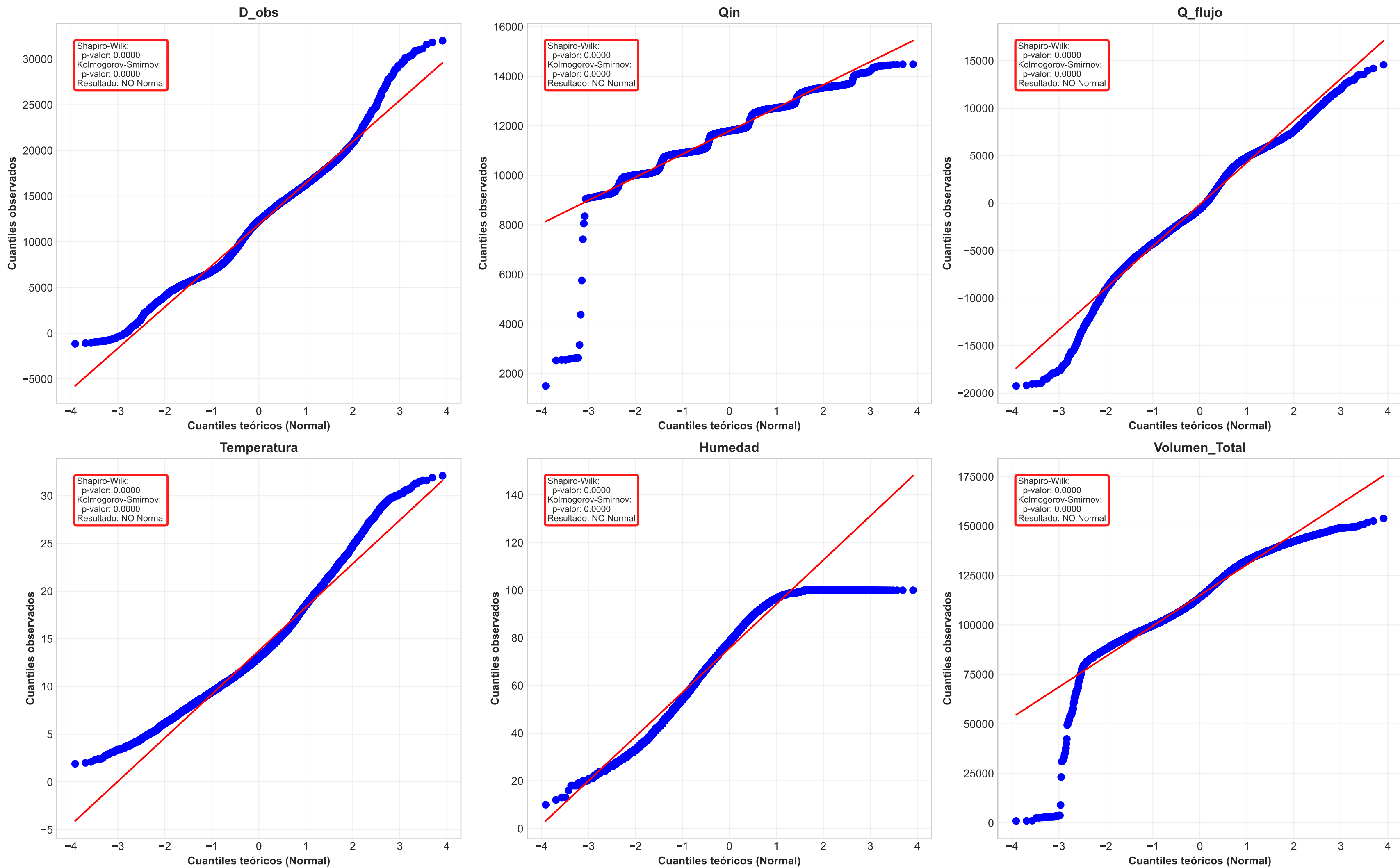
Figura 4.8: Análisis de Normalidad - Q-Q Plots y Tests Estadísticos (Justificación de uso de métodos no paramétricos y modelos ML robustos)
