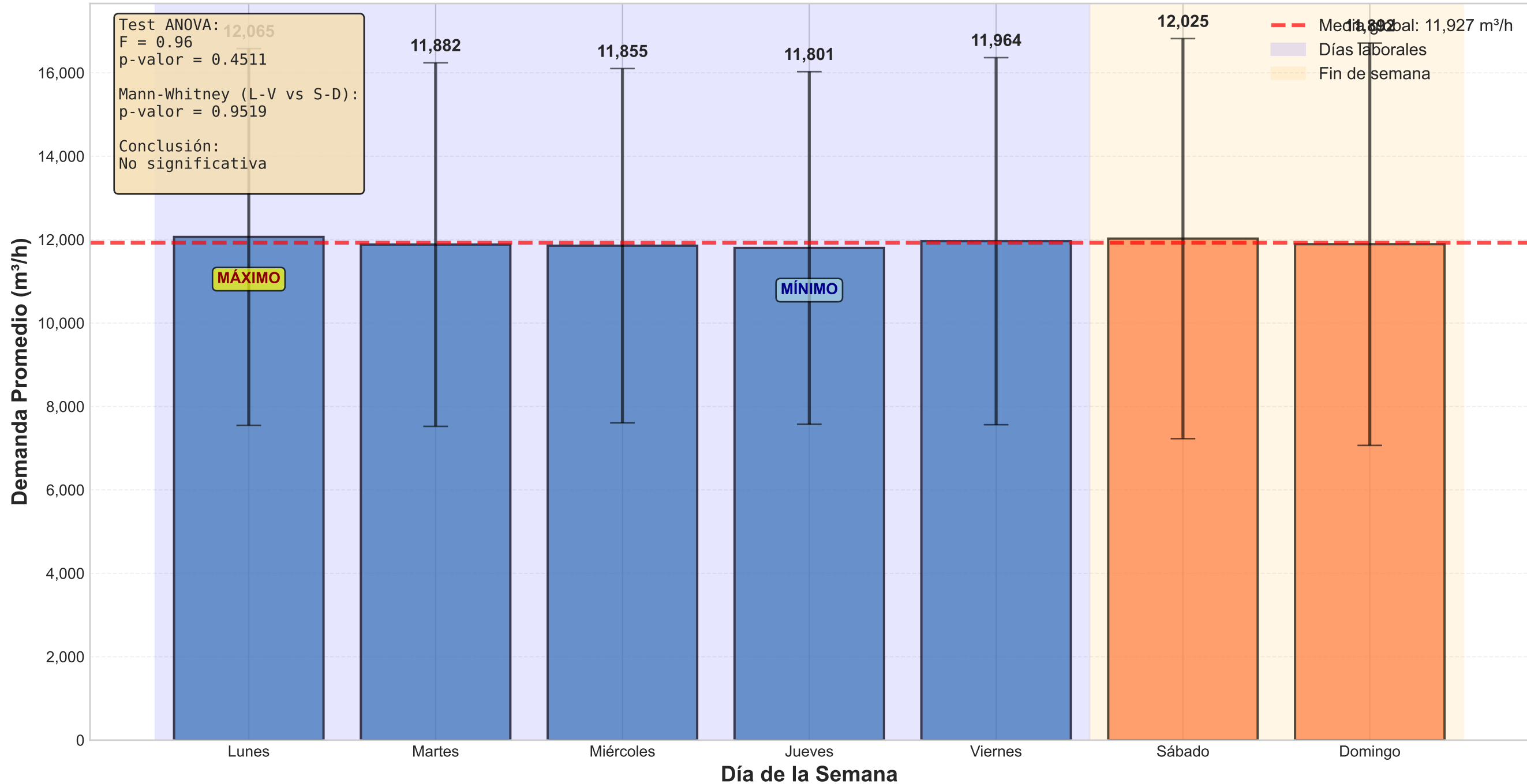
Figura 4.1.3: Ciclo Semanal de Demanda de Agua Potable - Gran Valparaíso Demanda promedio por día (N = 14,882 horas, 620 días)
