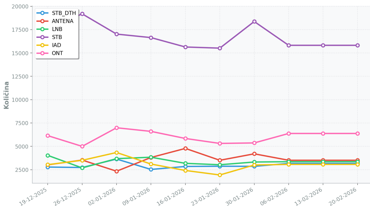
Trend ukupne CPE opreme po tipu (Zadnjih 10 sedmica)
