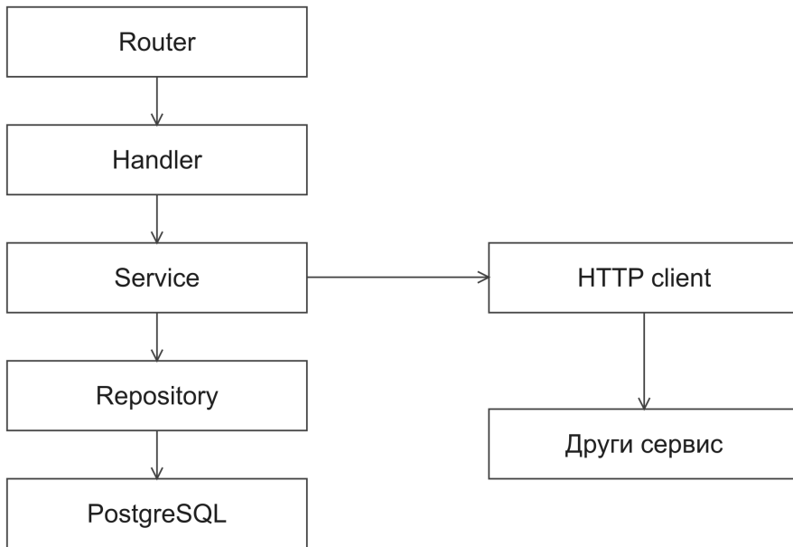
Слика 7: Слојеви обраде захтева у серверском сервису
