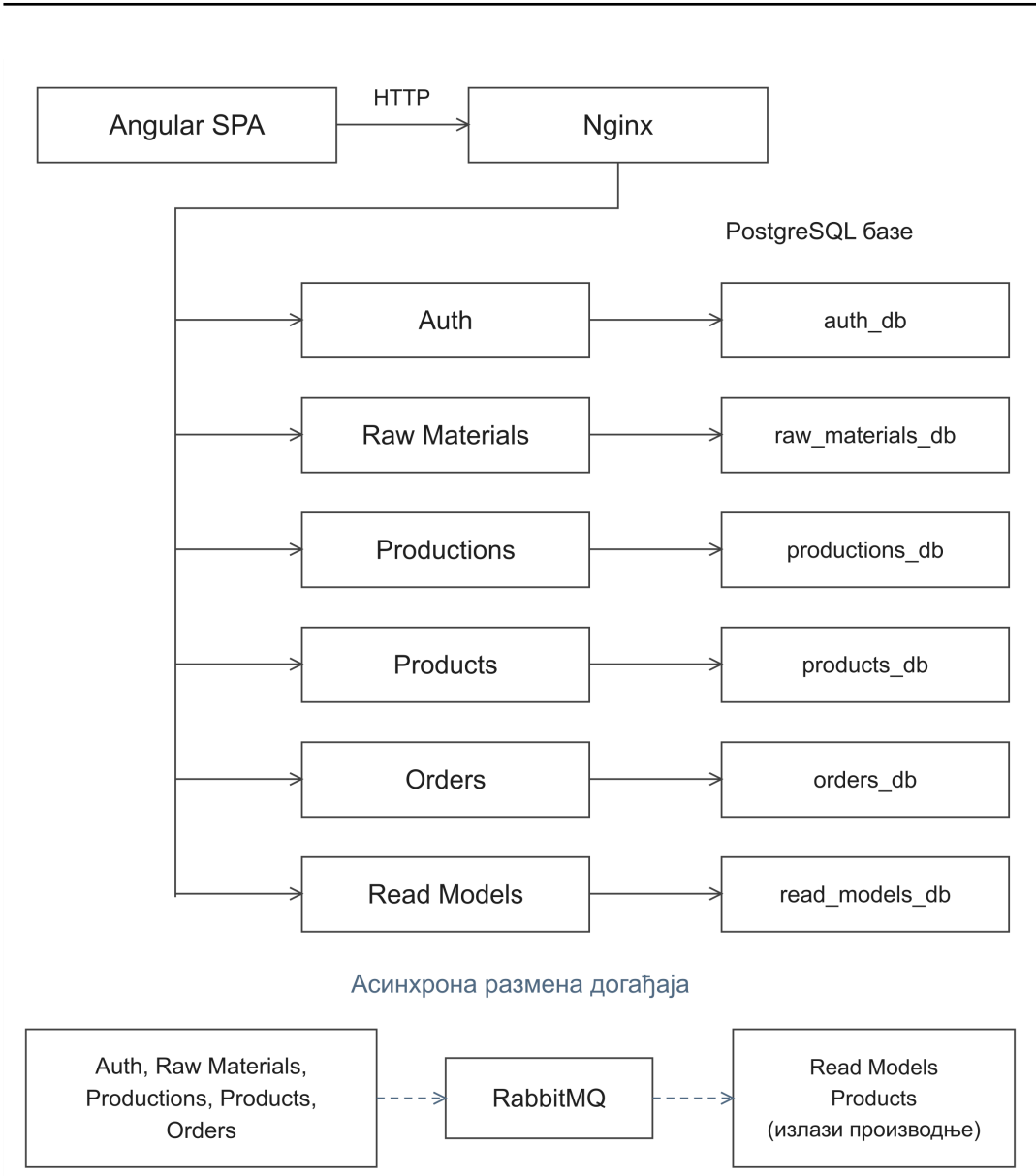
Слика 6: Логички преглед архитектуре платформе LocalBite
