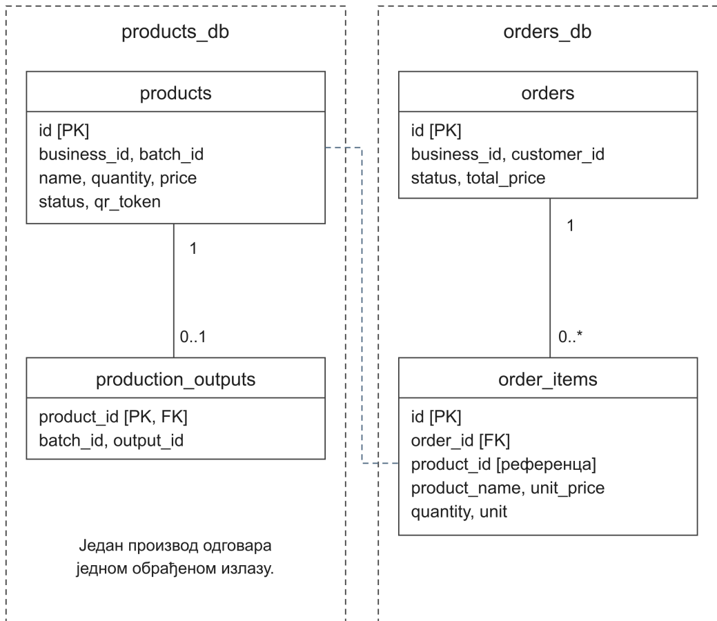
Слика 11: Основни модел производа и поруџбина са границама база
