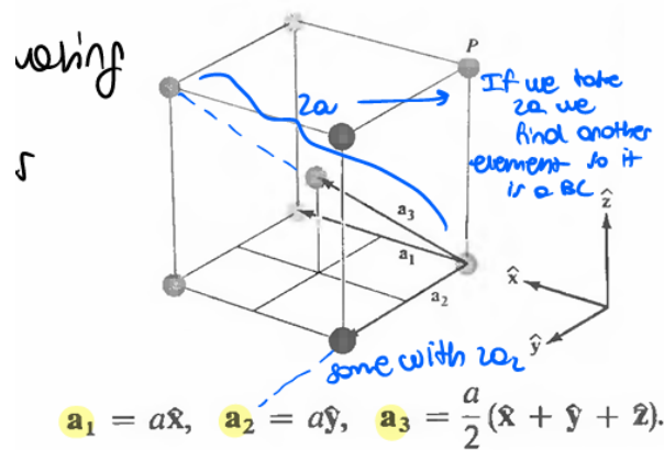
Figura 2.7: Prendendo due volte il vettore a_3 incontro un atomo del cristallo quindi è per questo che è un reticolo di Bravais
