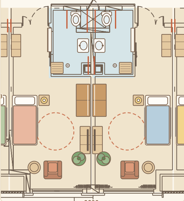
标准居室平面 (201-202 镜像)
