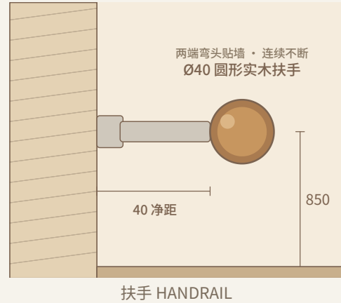
扶手 HANDRAIL
