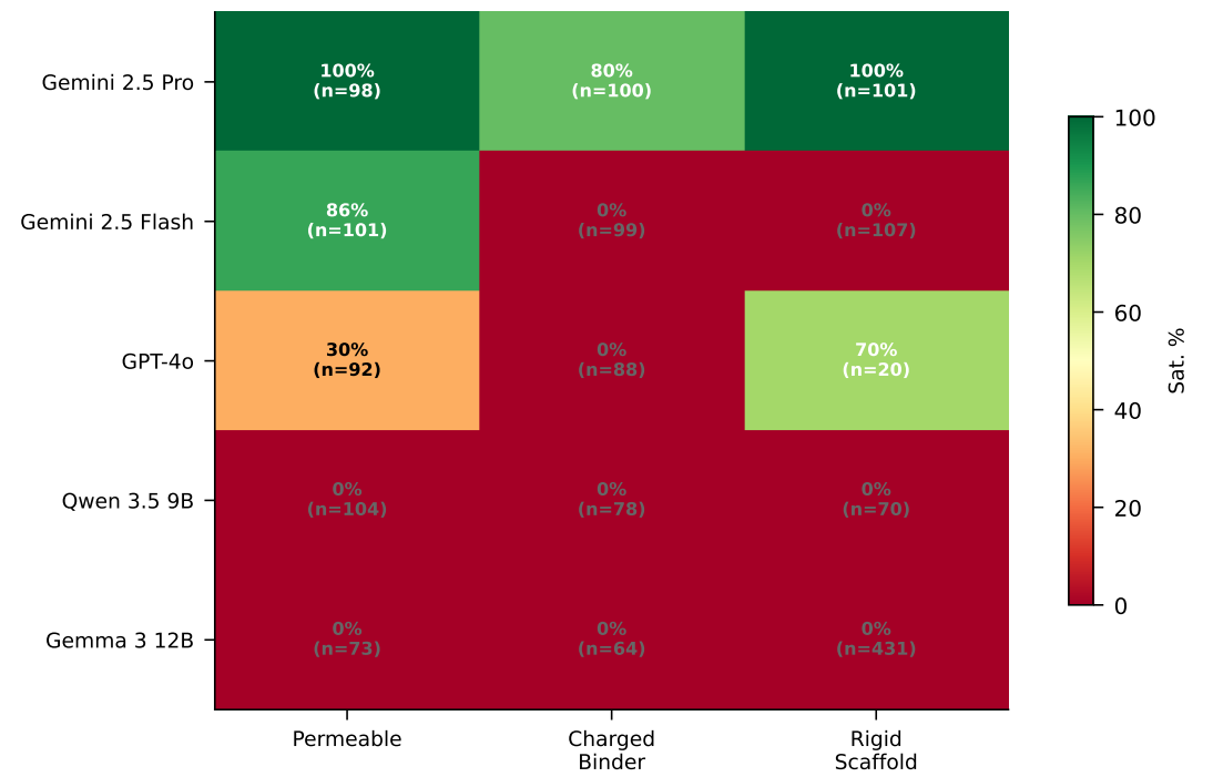
(d) Constraint Satisfaction
