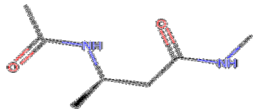
β-amino acid (β-alanine analog)
