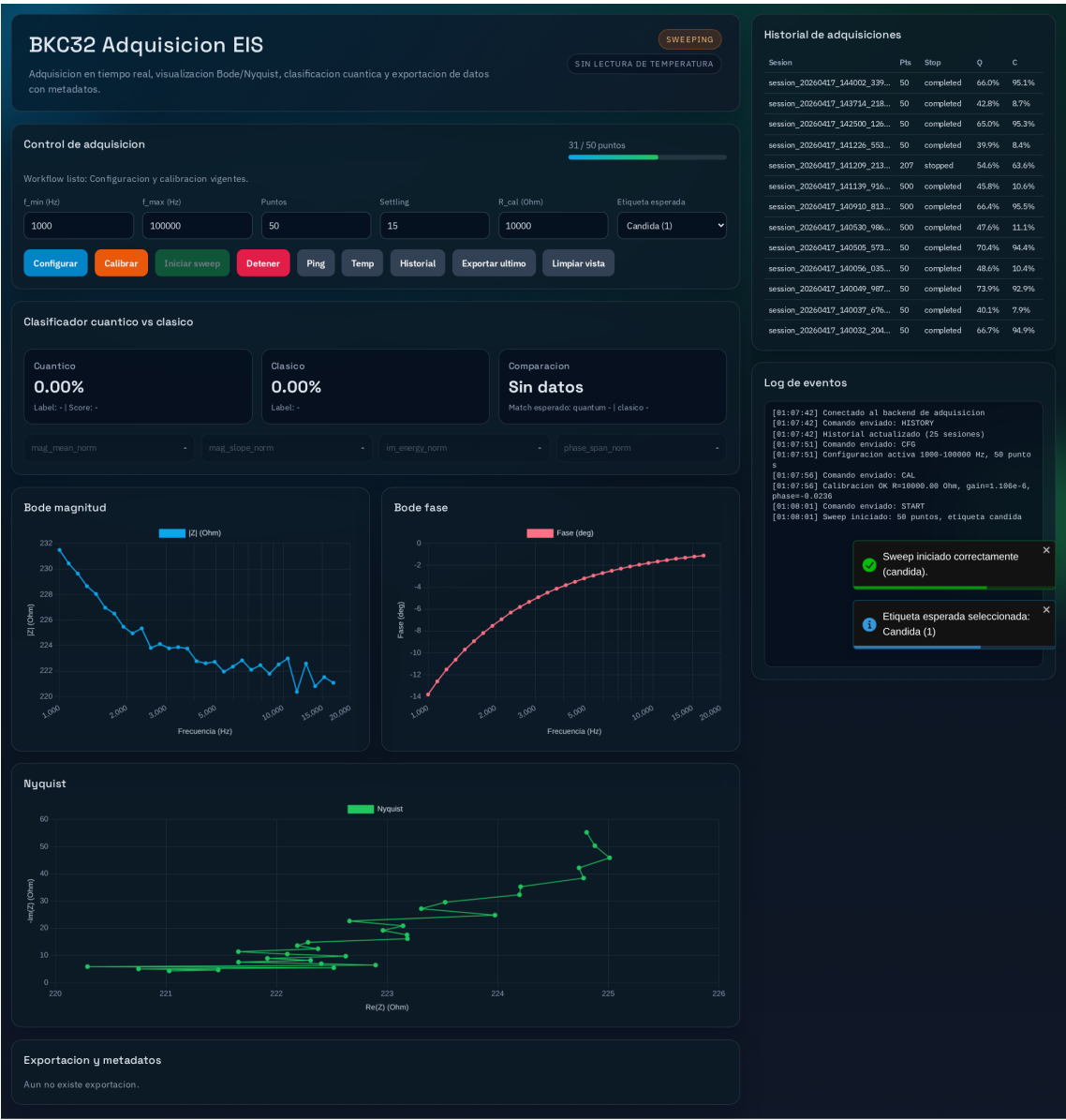
Figura 4.5: Interfaz durante la ejecución de un barrido (31/50 puntos), con actualización en vivo de Bode de magnitud, Bode de fase y Nyquist. Fuente: elaboración propia.
