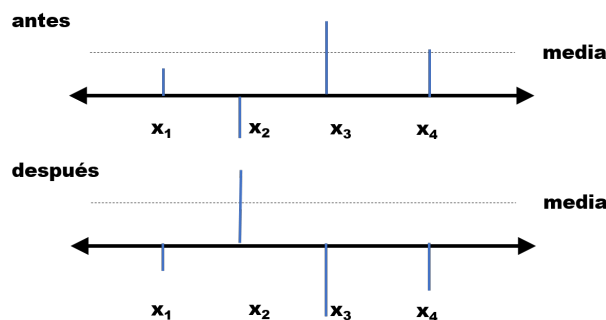
Figura 4.1: Inversión sobre la media del algoritmo de Grover. El conjunto de x_i son las amplitudes de cada estado cuántico. La línea discontinua es la media de las amplitudes. Después de cada inversión, la amplitudes grandes se vuelven más grandes y las pequeñas más pequeñas. Fuente: elaboración propia
