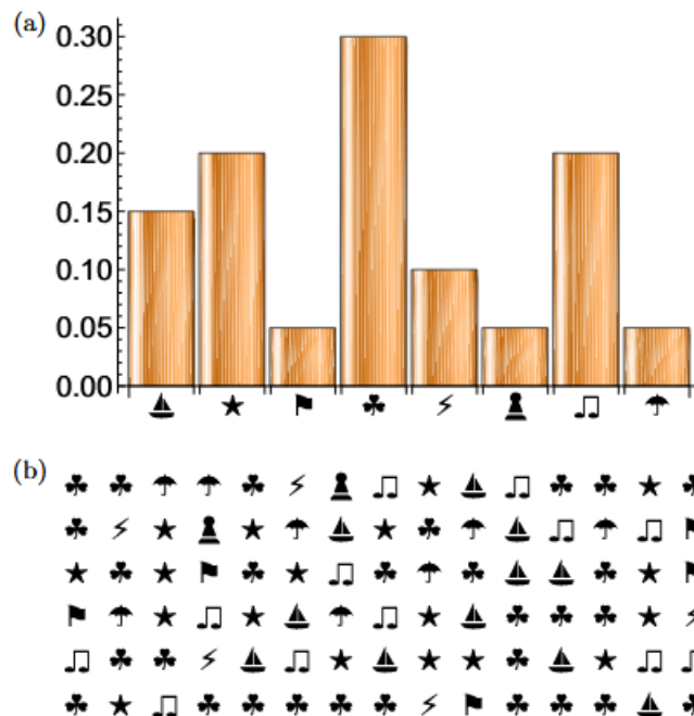
Figura 4.2: a) Un ejemplo de distribución de probabilidad sobre 8 símbolos. (b) 100 muestras aleatorias de la distribución de probabilidad. El objetivo de un problema de muestreo es calcular muestras como las secuencias mostradas en (b) cuya complejidad puede ser diferente a la complejidad de calcular la distribución de probabilidad (a). Fuente: Lund (2017)
