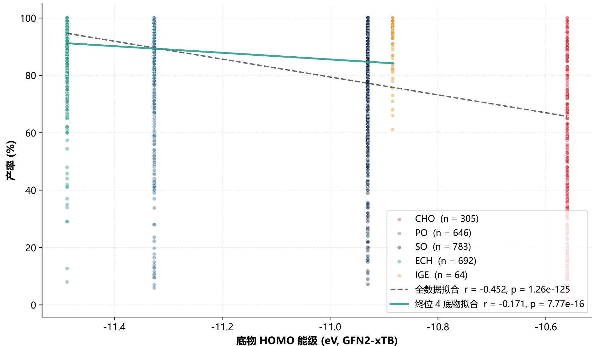
图 5. 底物 HOMO 能级 vs 产率: CHO 拉低整体相关性
