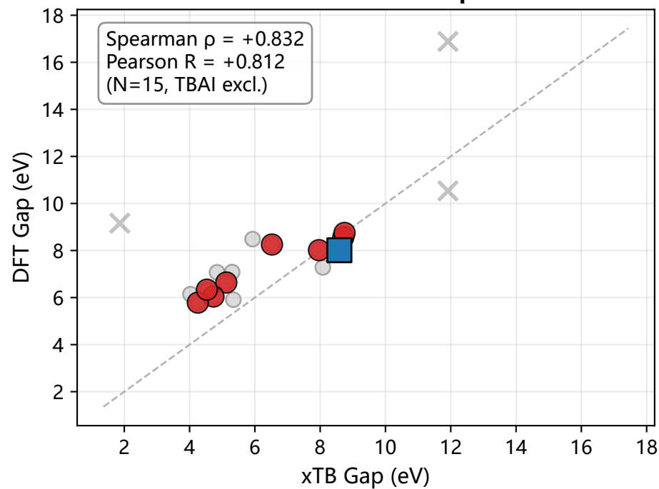
HOMO-LUMO Gap
