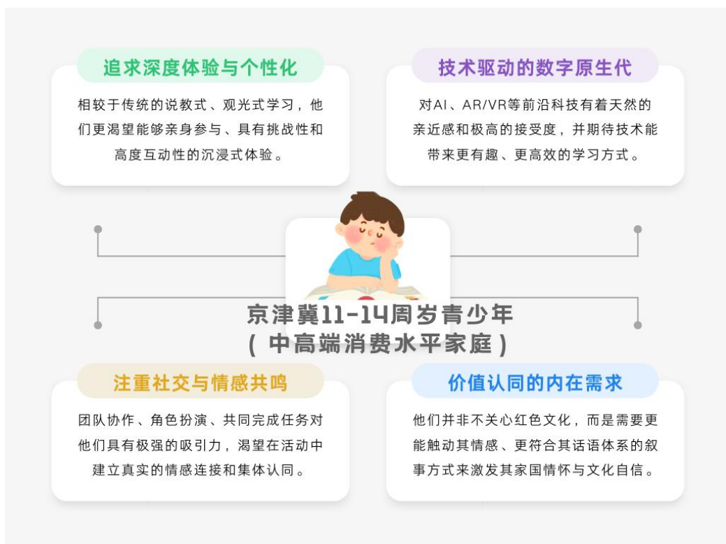
图2-1 用户画像图
