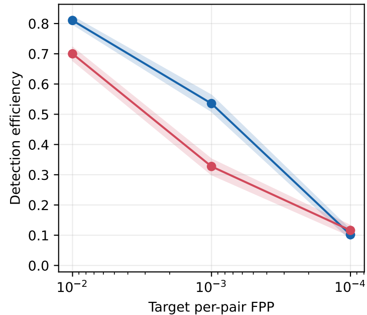
SIS
