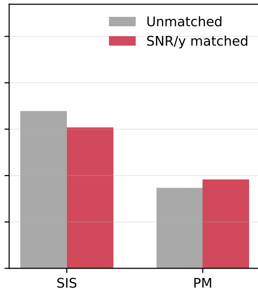
CQT-DeiT
