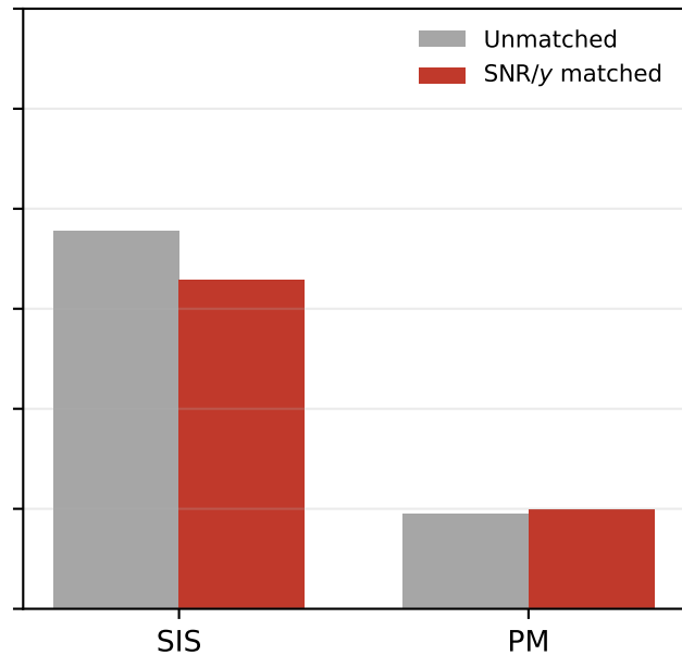
CQT-DeiT
