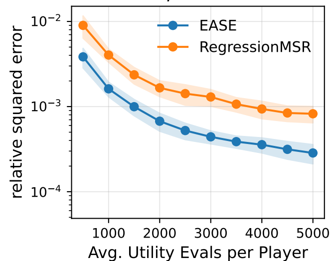
(d) EASE vs RegressionMSR, \eta = 0.5
