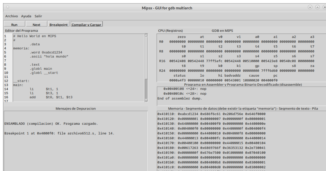
Figura 1: Interfaz visual del programa mipsx
