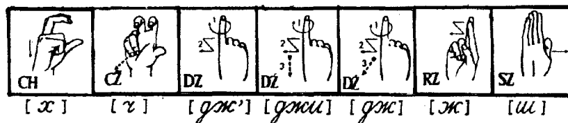
Рис. 9. Польские дактилемы
