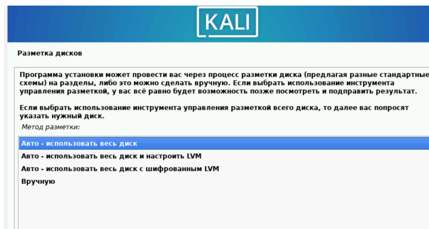
Рис. 4.13: Разметка дисков
