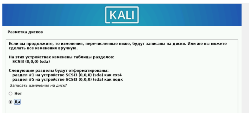
Рис. 4.17: Разметка дисков
