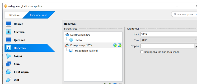
Рис. 4.20: Проверка носителей
