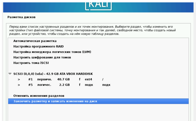
Рис. 4.16: Разметка дисков
