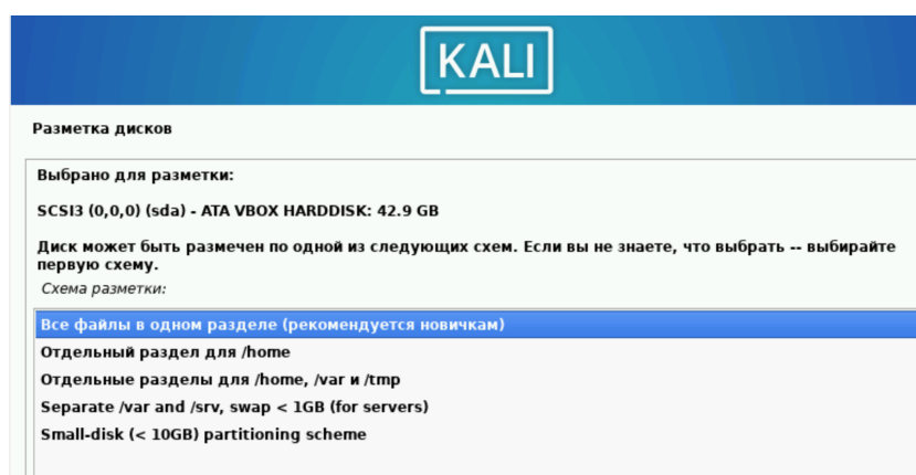
Рис. 4.15: Разметка дисков
