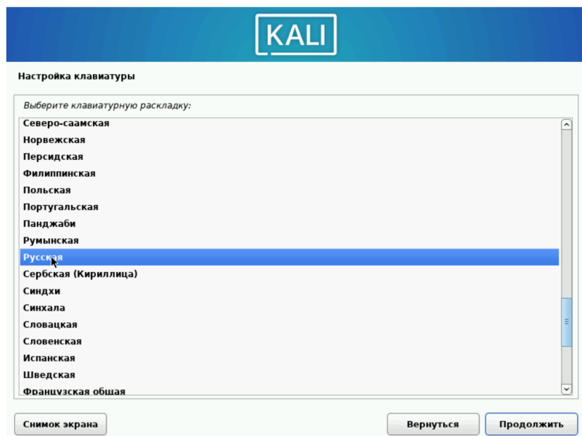
Рис. 4.6: Настройка клавиатуры
