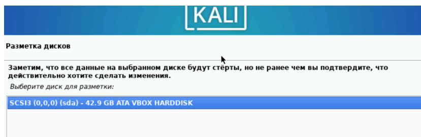
Рис. 4.14: Разметка дисков
