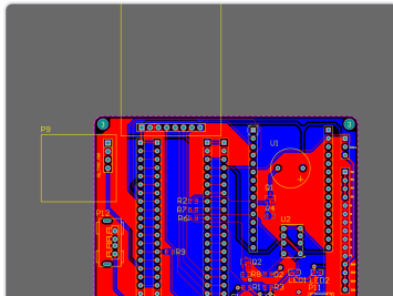
智能空气检测器 PCB
