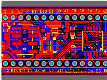
STM32 核心板 PCB
