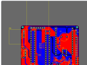
智能空气检测器 PCB
