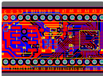
STM32 核心板 PCB
