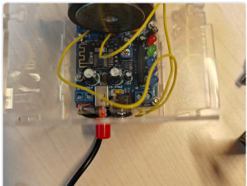
蓝牙音箱
