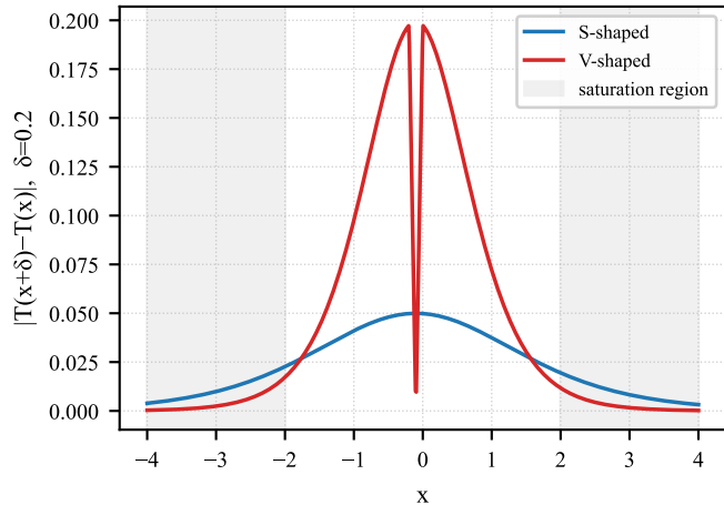
Leverage (washout)
