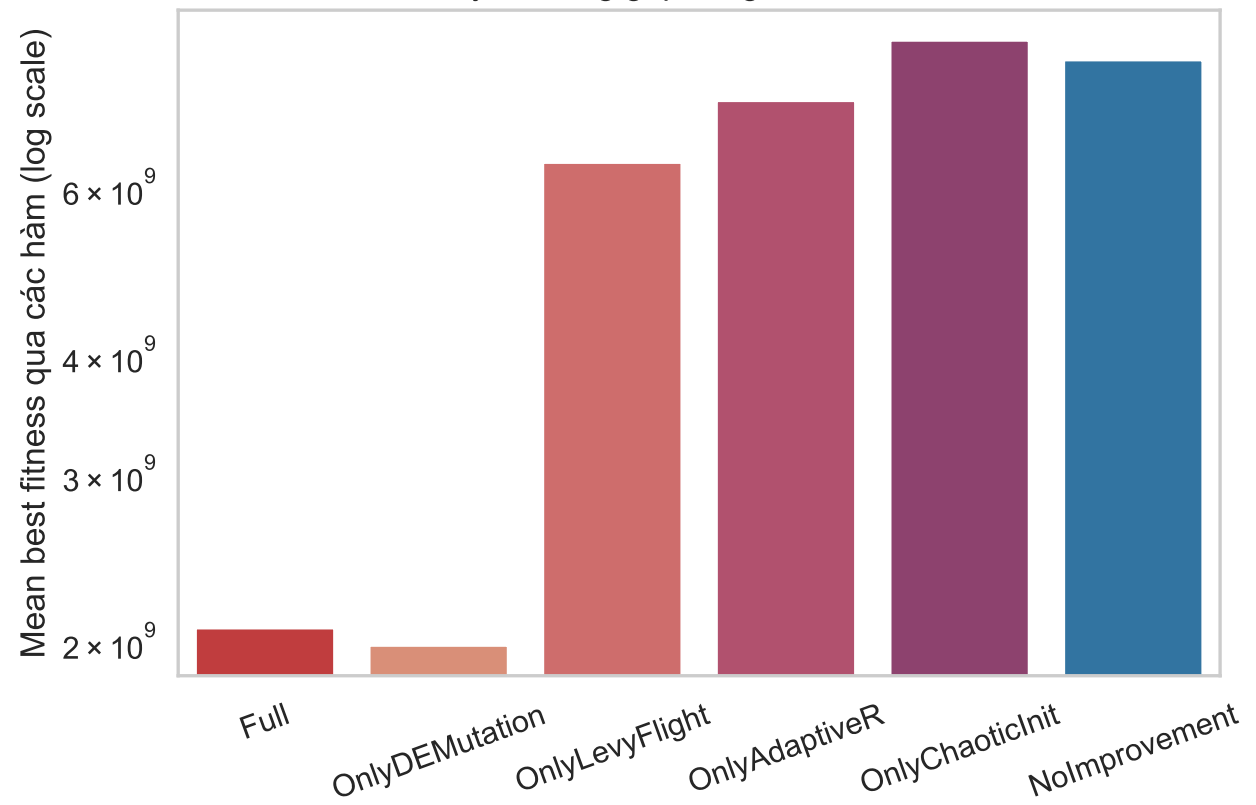
Ablation study — đóng góp từng cải tiến của ECL-SCSO
