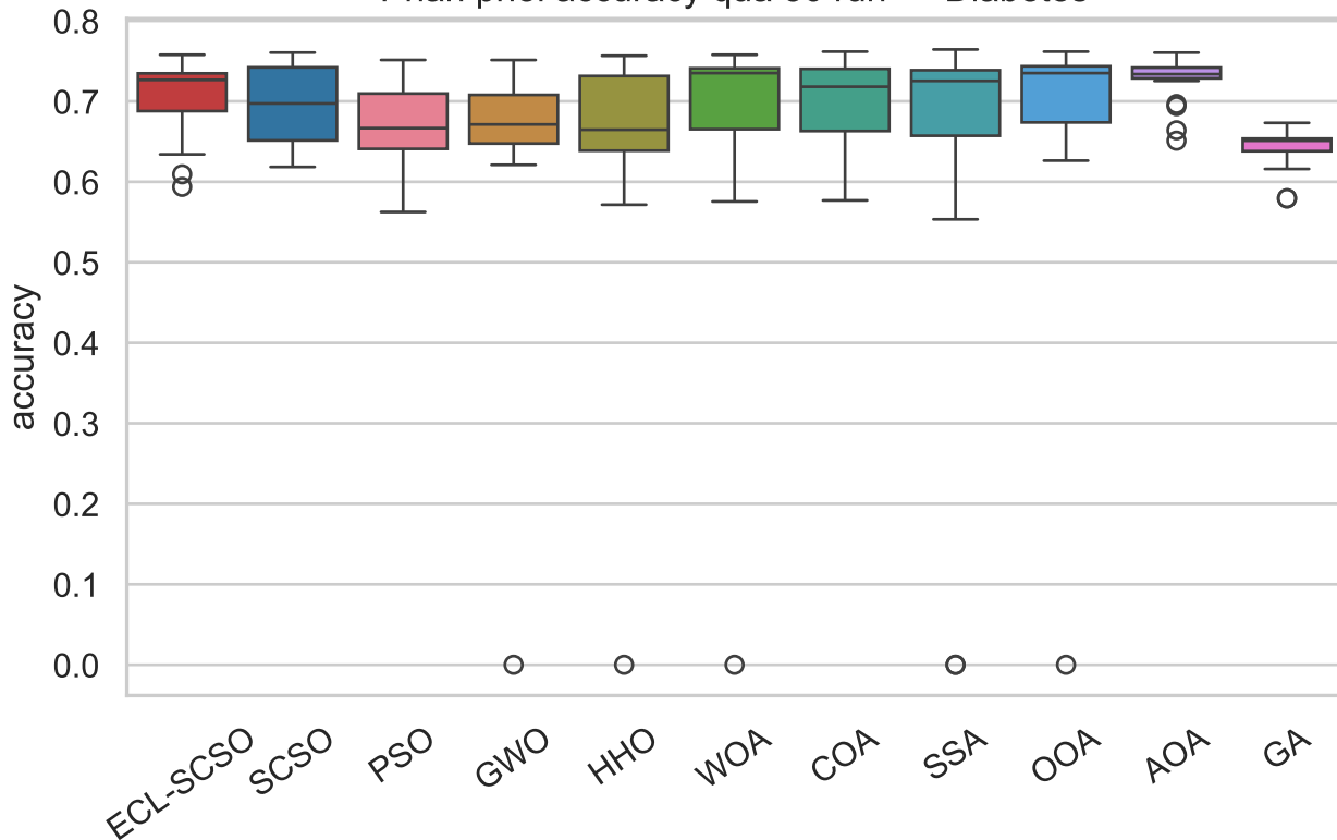
Phân phối accuracy qua 30 run — Diabetes
