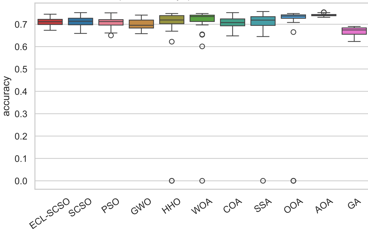
Phân phối accuracy qua 30 run — GermanCredit
