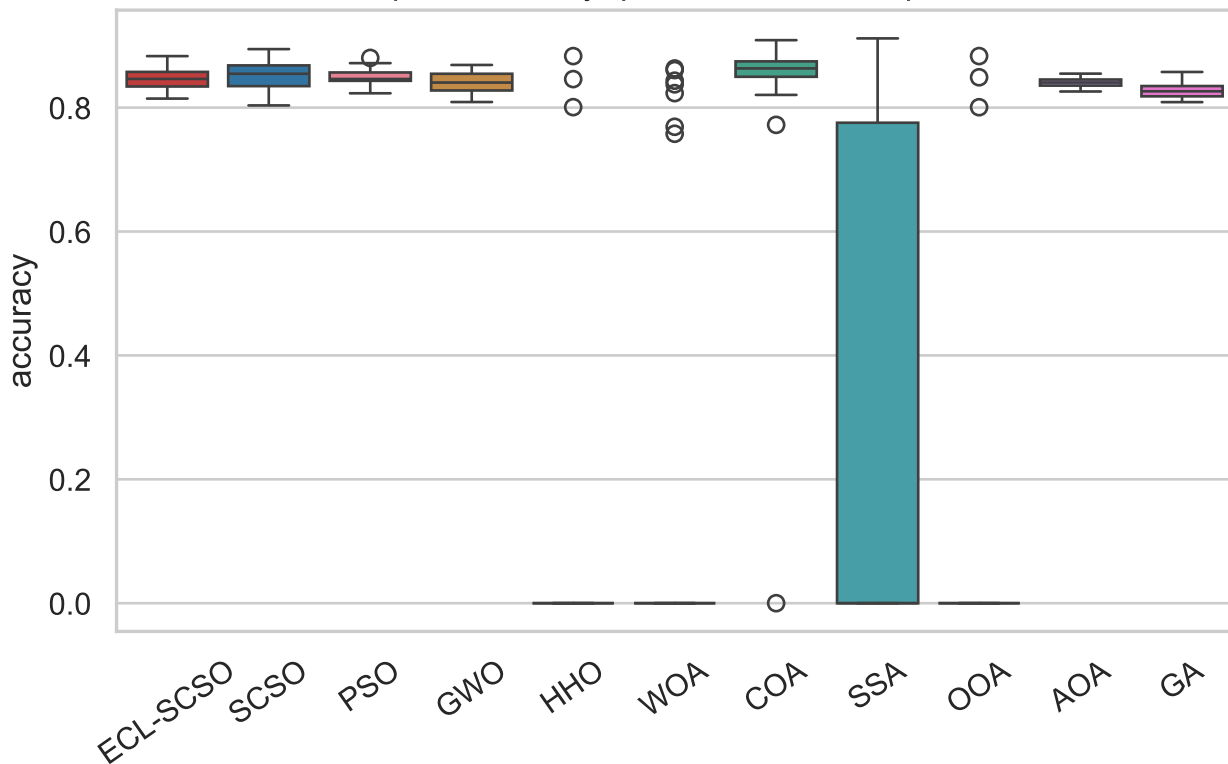
Phân phối accuracy qua 30 run — IonosphereEW
