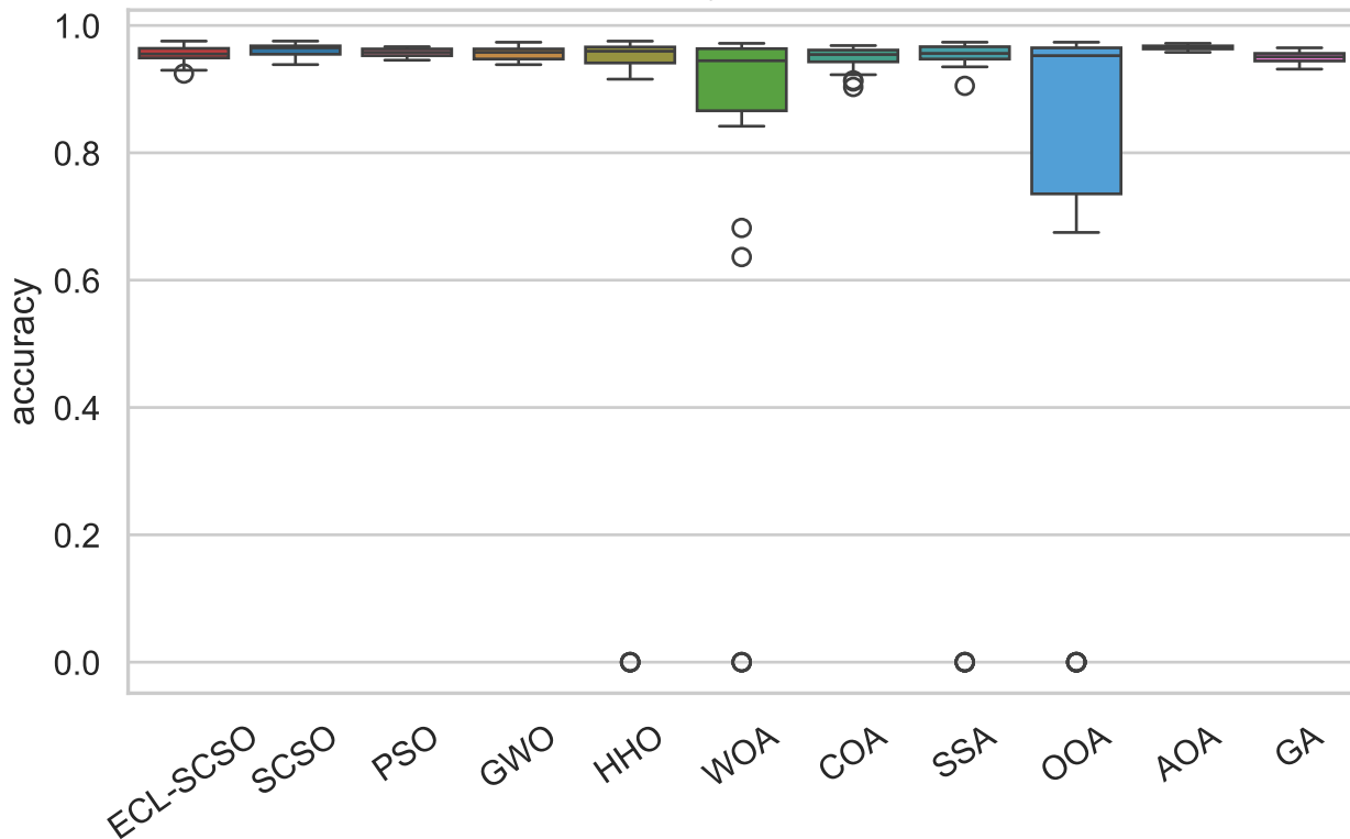
Phân phối accuracy qua 30 run — WDBC
