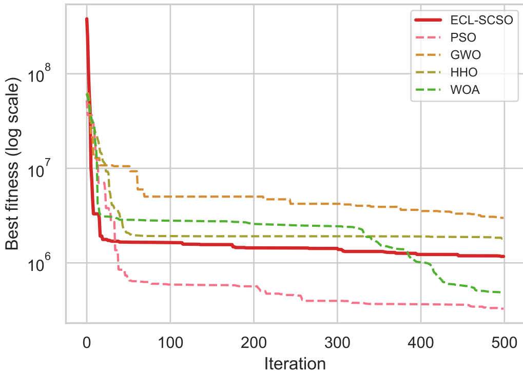
CEC2017_F13
