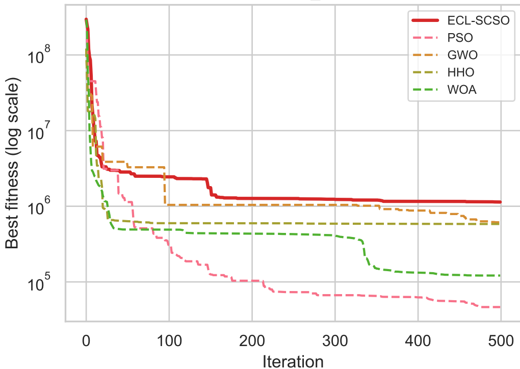
CEC2017_F17
