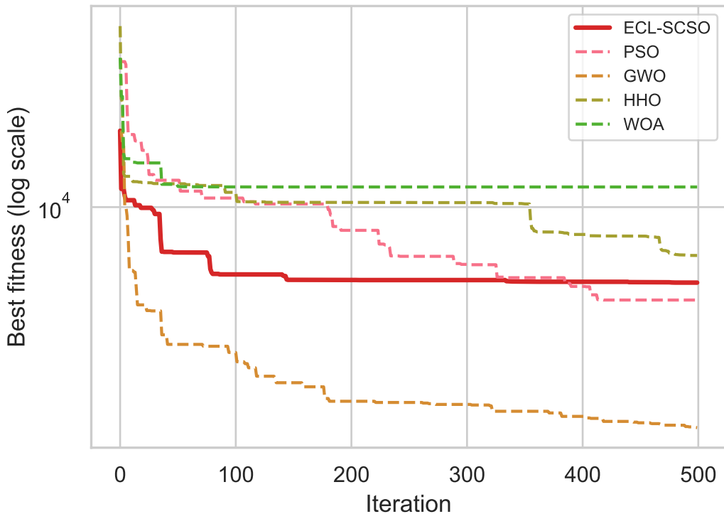
CEC2017_F19
