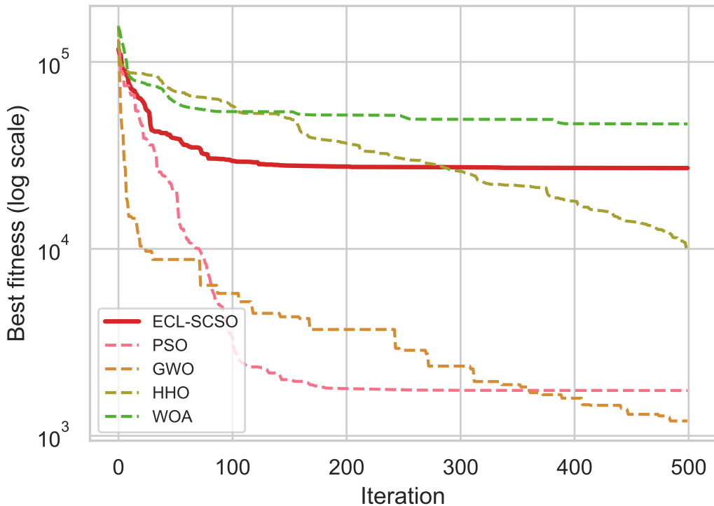
CEC2017_F4
