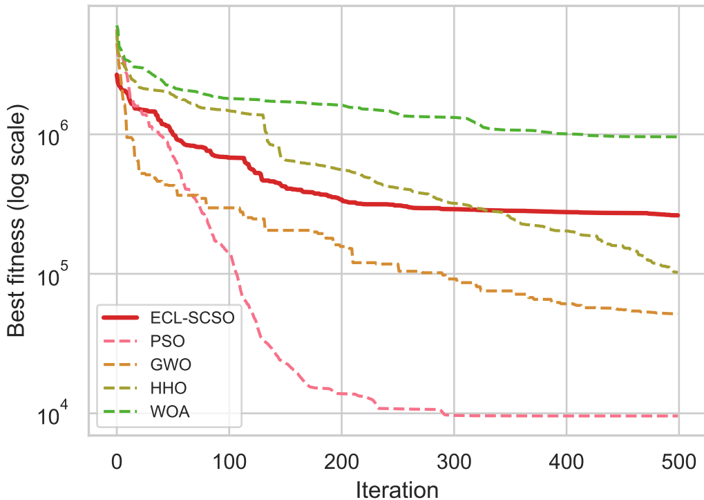
CEC2017_F6
