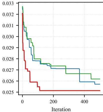
WDBC
