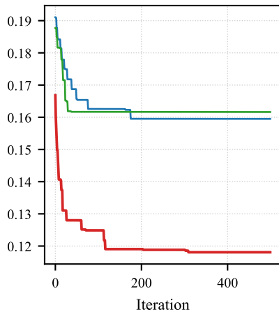
ColonCancer
