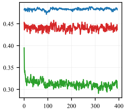
WDBC
