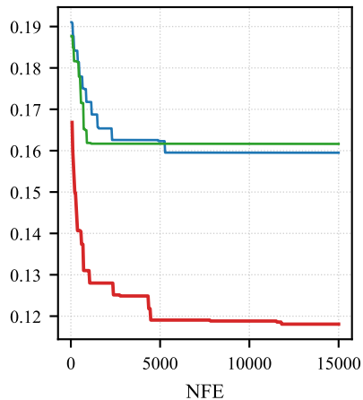
ColonCancer
