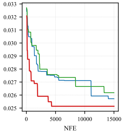
WDBC
