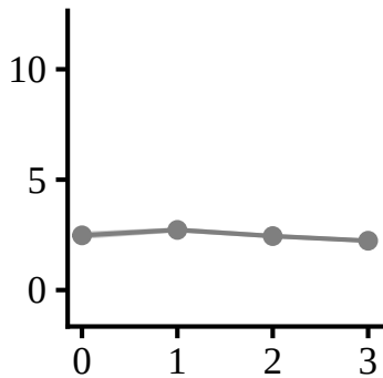
AtP*
