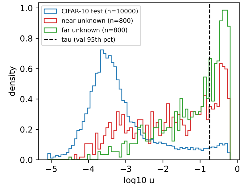
MSP: 1 - max softmax
