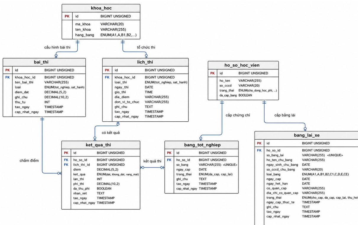
Hình 3.8 Sơ đồ ERD - Phân hệ thi cử và bằng cấp
