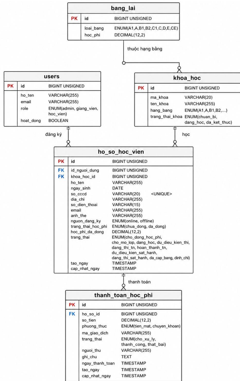
Hình 3.6 Sơ đồ ERD - Phân hệ hồ sơ học viên và học phí
