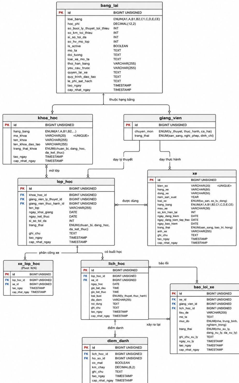
Hình 3.7 Sơ đồ ERD - Phân hệ đào tạo
