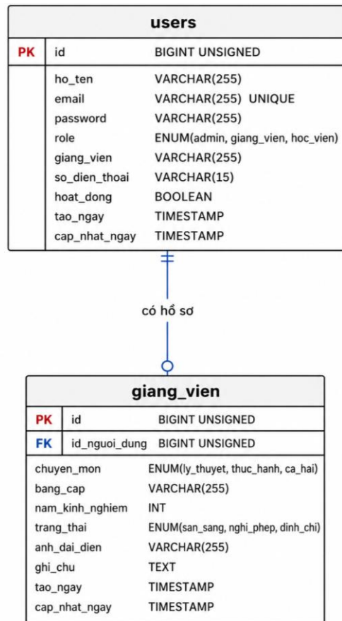
Hình 3.5 Sơ đồ ERD - Phân hệ tài khoản và nhân sự
