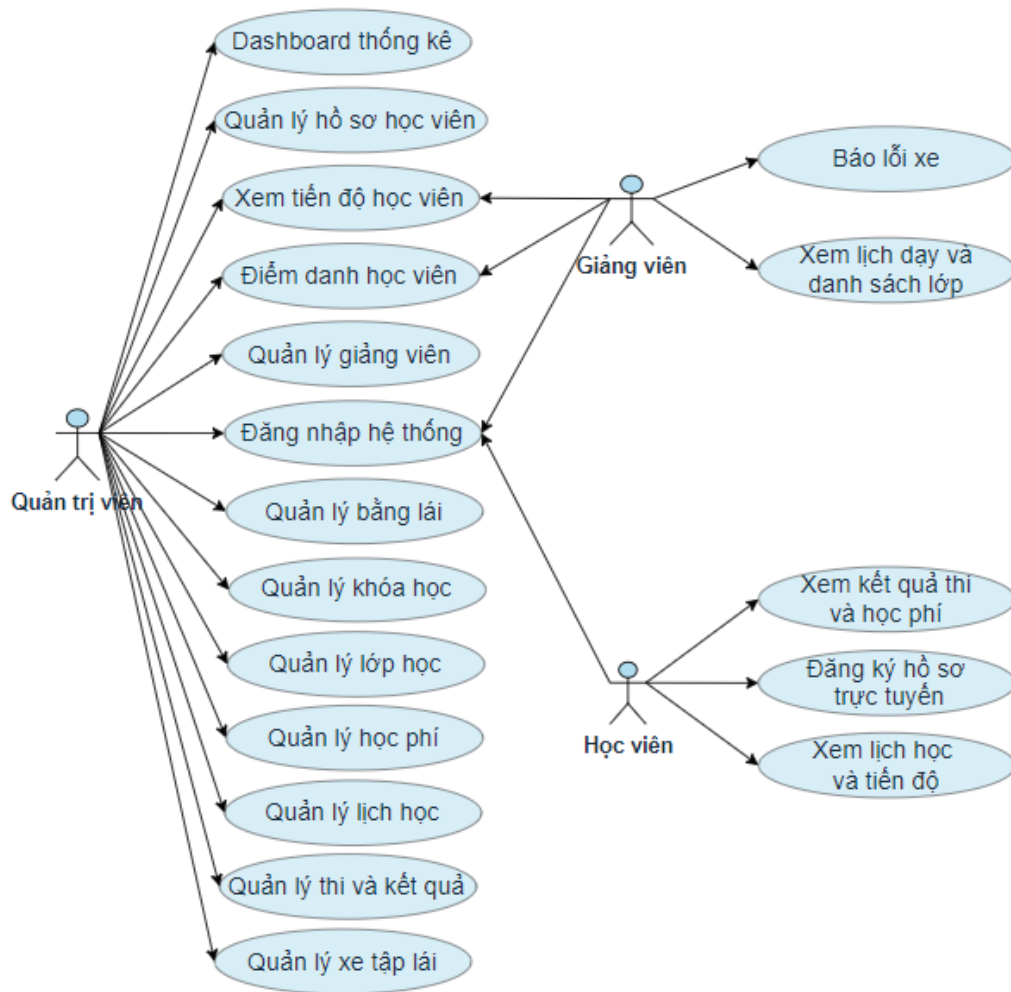
Hình 3.1 Biểu đồ use case tổng quát
