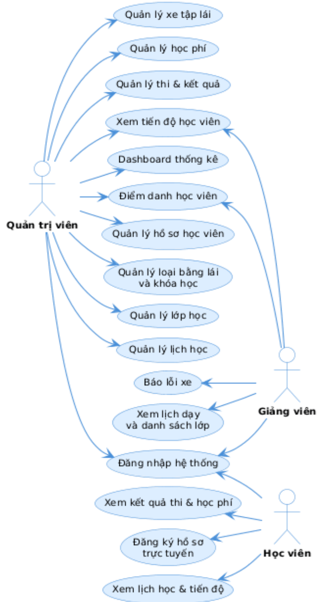
Hình 3. 1 Biểu đồ use case tổng quát
