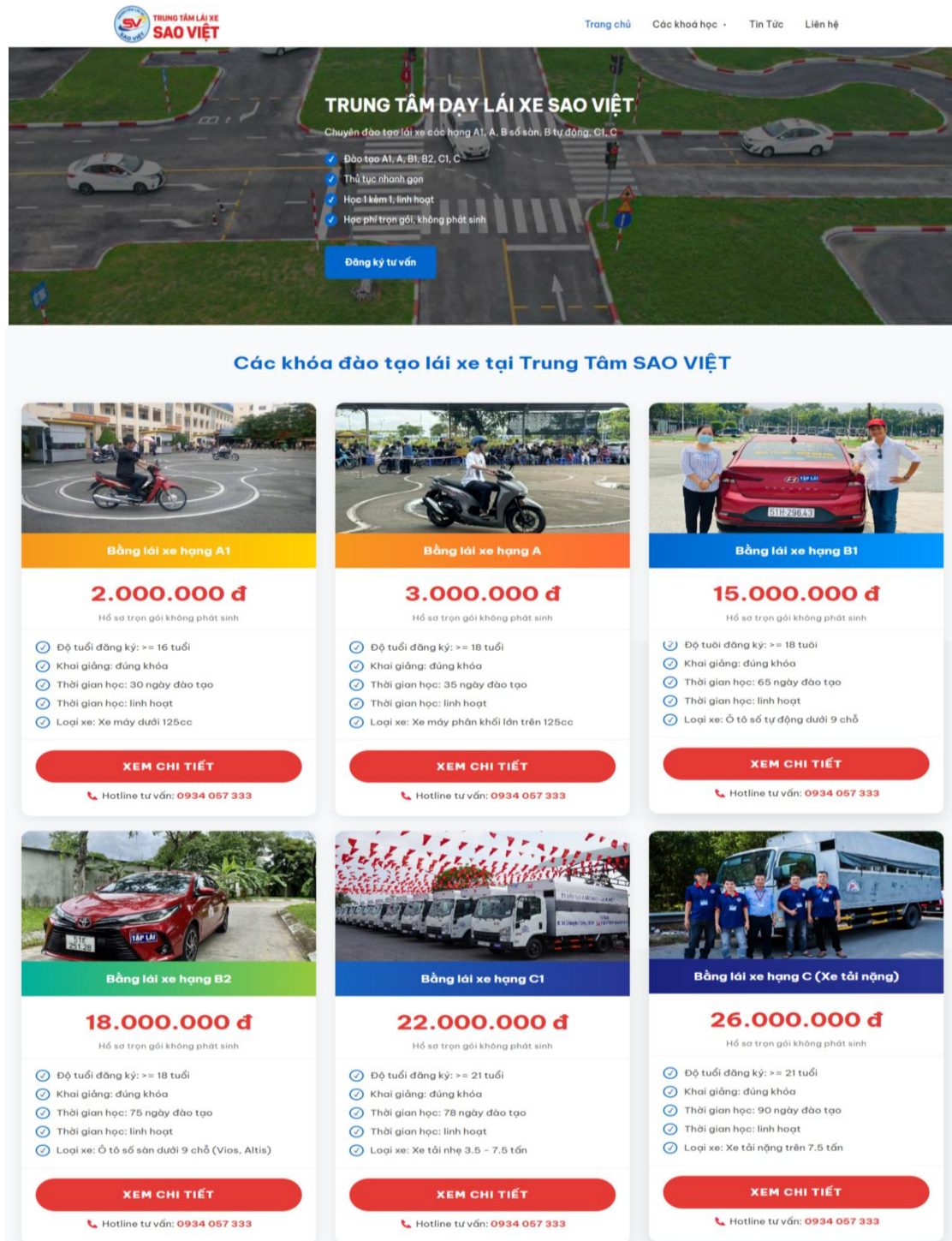
Hình 4.1 Trang chủ
