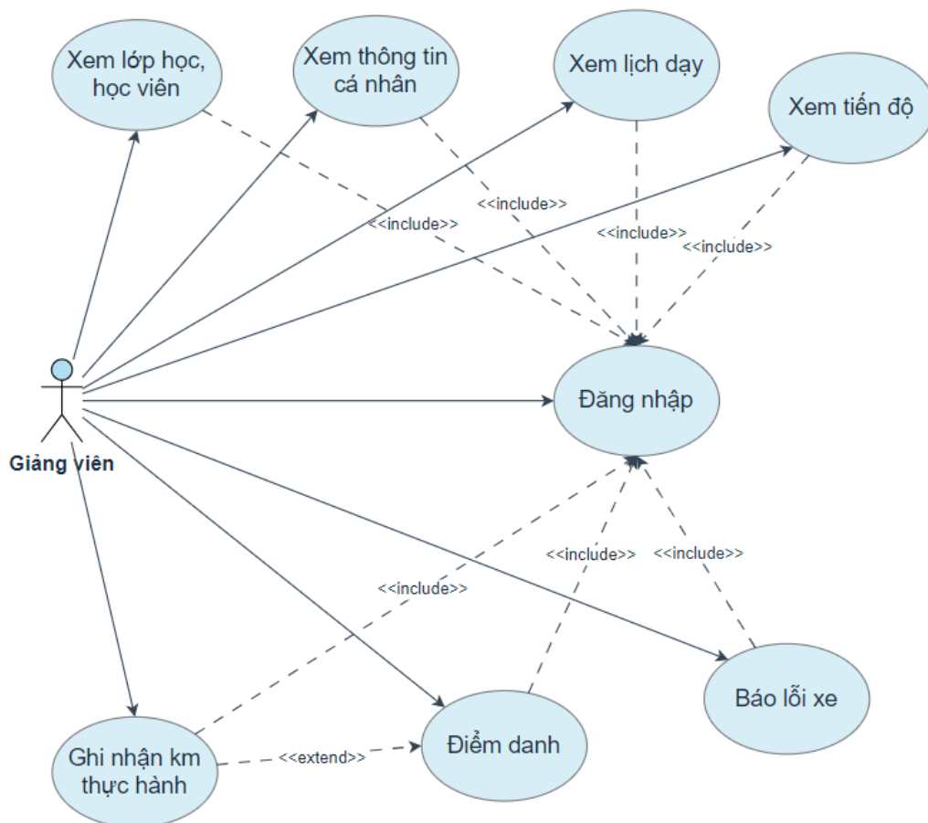
Hình 3. 3 Biểu đồ use case giảng viên
