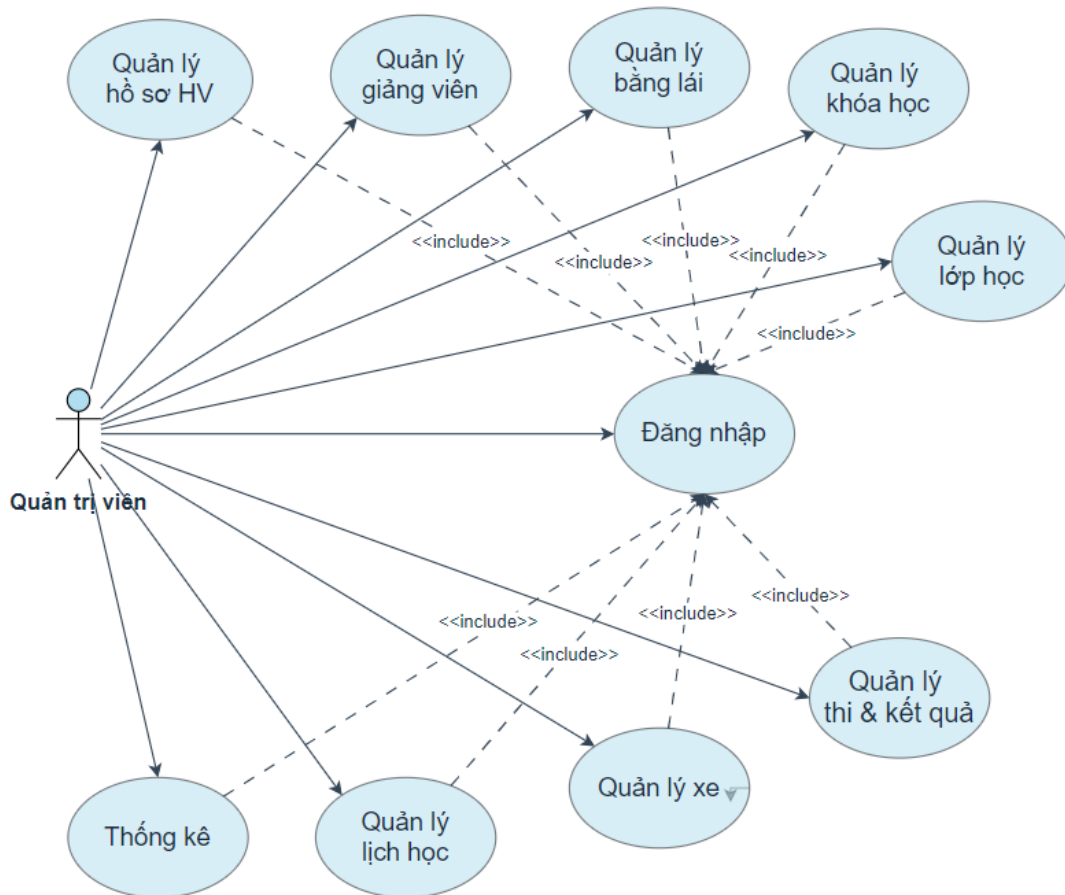
Hình 3. 2 Biểu đồ use case quản trị viên
