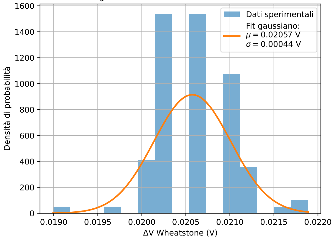
Istogramma della tensione di Wheatstone
