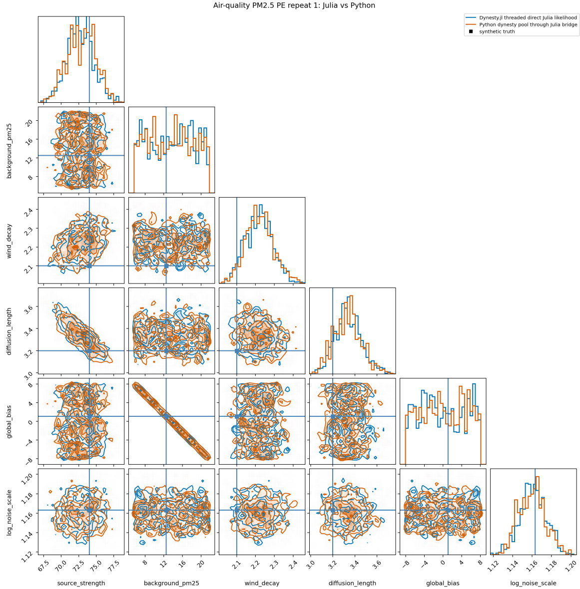
图 4: 真实空气质量 PM2.5 PE posterior overlay。蓝色为 Dynesty.jl threaded direct Julia likelihood; 橙色为 Python dynesty pool through Julia bridge; 黑色 marker 为 synthetic truth。
